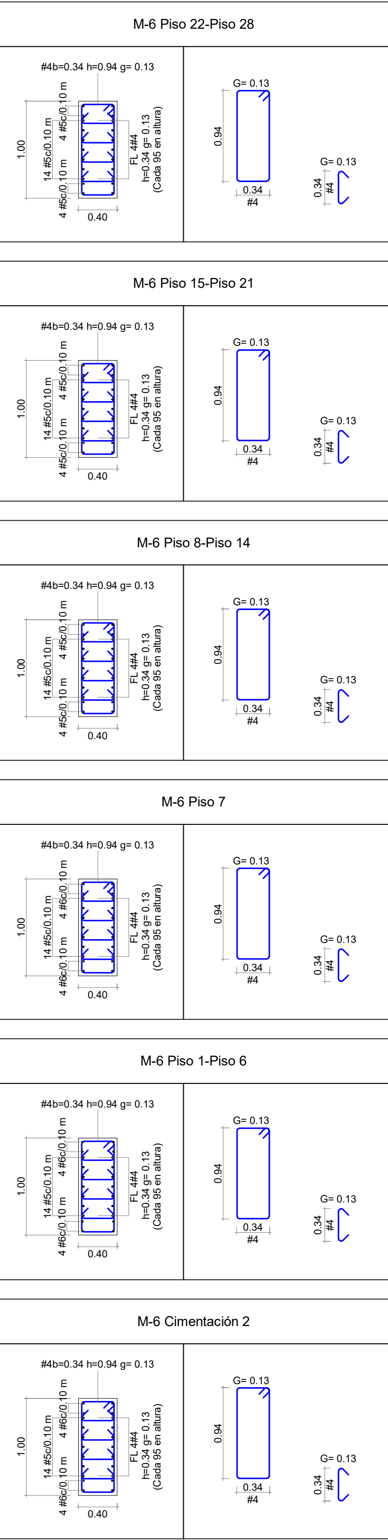
DETALLE SOBRE ANCHO EN MURO M-6 Escala 1 : 25
